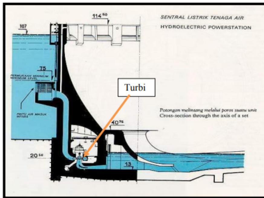
Gambar 8. Prinsip/Cara Kerja PLTA
